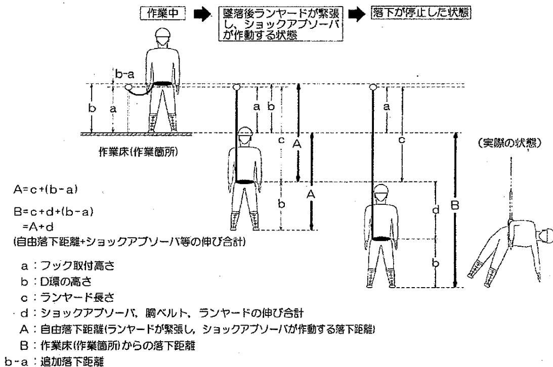
図2 胸ベルト型の落下距離等
